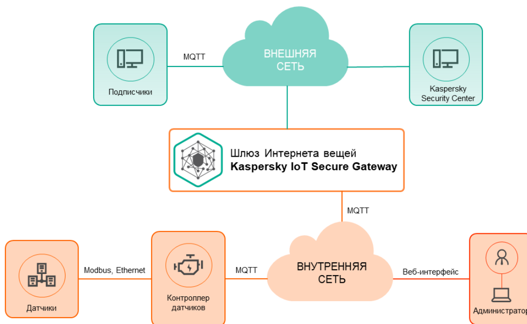
Типовая схема развертывания Kaspersky IoT Secure Gateway
